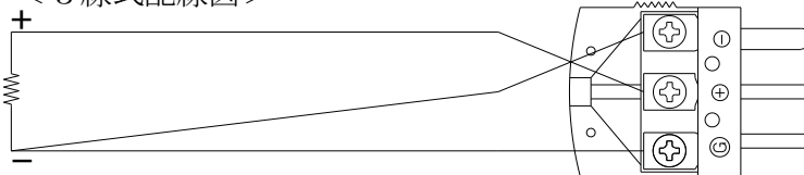
< 3線式配線図 >
