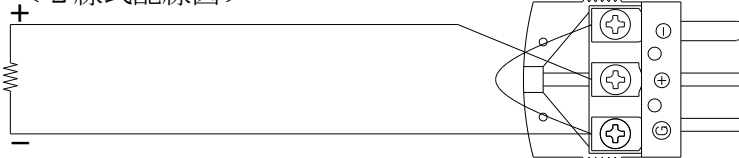
< 2線式配線図 >
